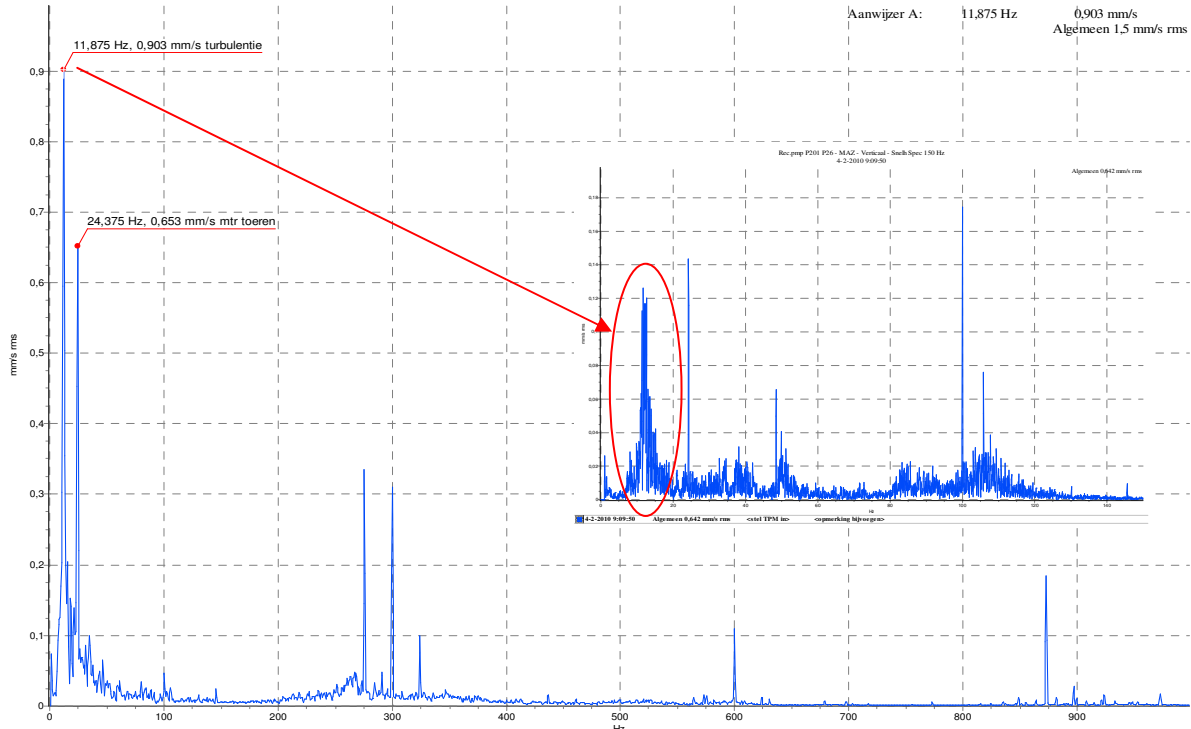
Rec.pmp P201 P26 - Axiaal Verticaal - Verticaal - Snelh Spec 1000 Hz 4-2-2010 9:11:03
