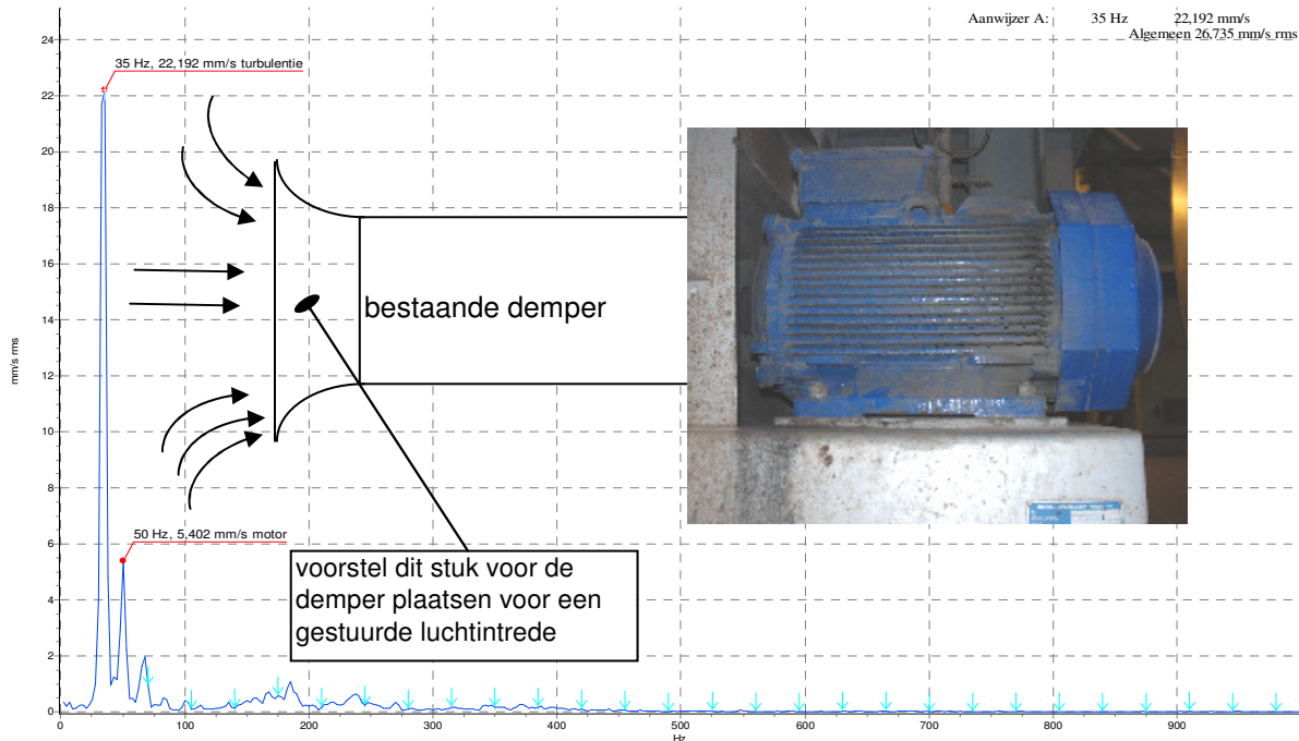
V- licht K2 100 - MAX - Axiaal - Snelh Spec 1000 Hz 30-11-2009 10:09:08
