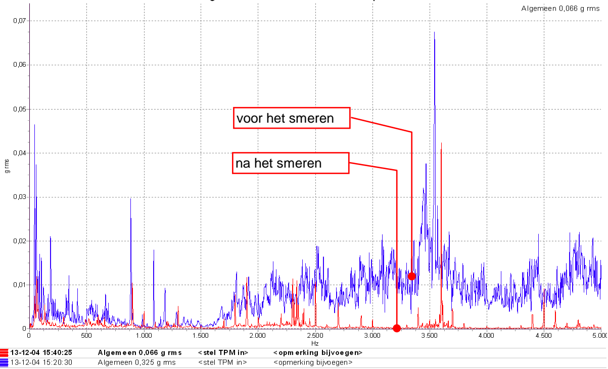
menger mixer - MAZ - Verticaal - Versn Freq 5000 Hz
