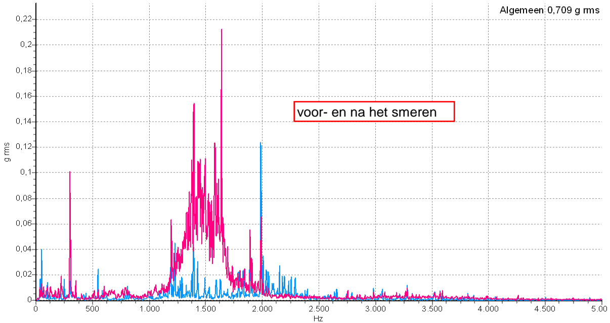
V- lucht K2 100 - MAZ - Verticaal - Versn Freq 5000 Hz
