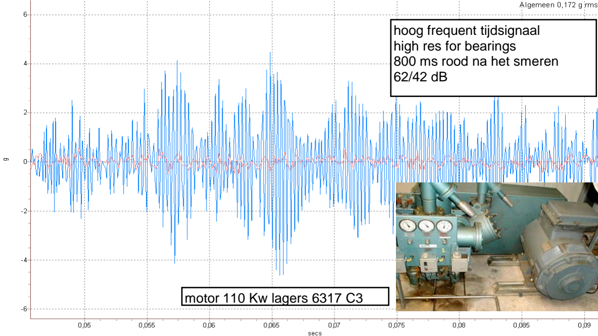
kCompres 2 onder - MAZ - Verticaal - Versn Tijd 800 ms
